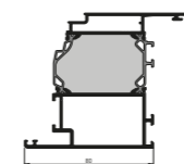
Flügelprofil 84/104 (SBN) 22207/22307 o. PU
