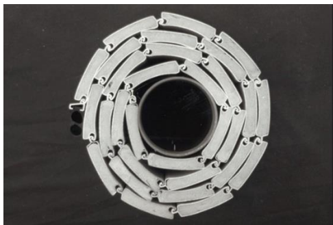
[heroal_1969_ausgeschäumter Rollladenstab]
