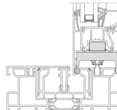
heroal S 65 HI s bezbariérovým prahem, s dodatečnou izolací a s HI těsněním, zobrazení v řezu
