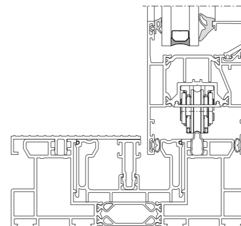
heroal S 65 s bezbariérovým prahem, bez dodatečné izolace a se standardními těsněními, zobrazení v řezu
